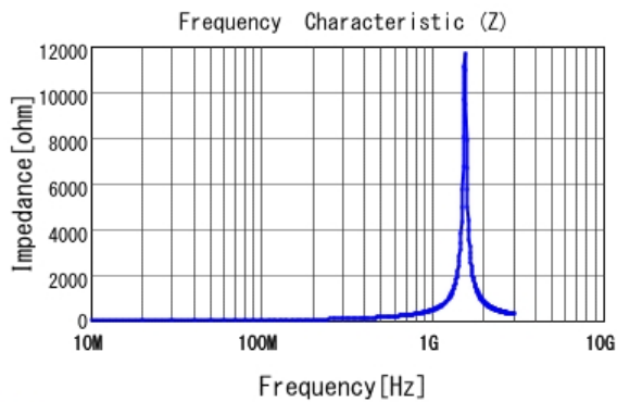
■ LQG15HN47NJ02 |Z|
