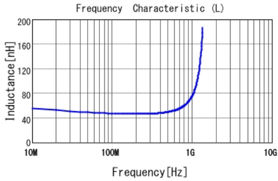
■ LQG15HN47NJ02 L
