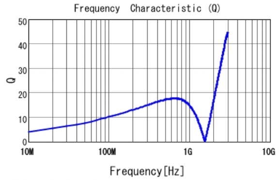
■ LQG15HN47NJ02 Q
