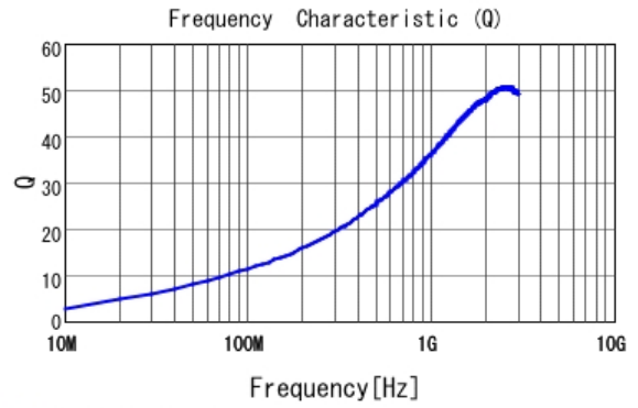
■ LQG15HN4N7S02 Q
