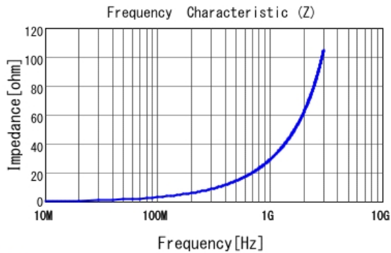
■ LQG15HN4N7S02 |Z|
