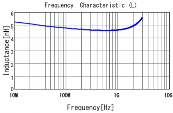
■ LQG15HN4N7S02 L
