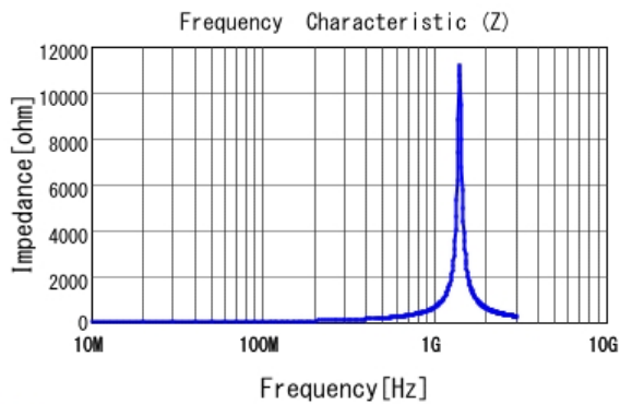
■ LQG15HN56NG02 |Z|
