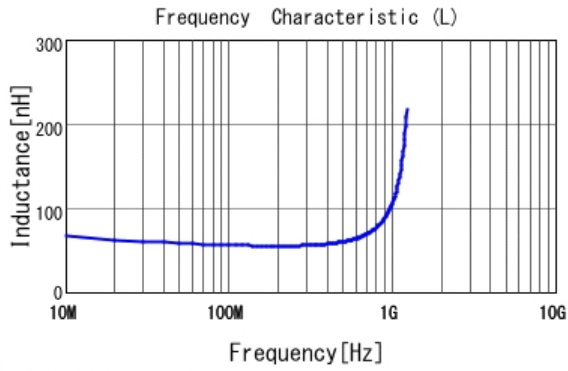
■ LQG15HN56NG02 L
