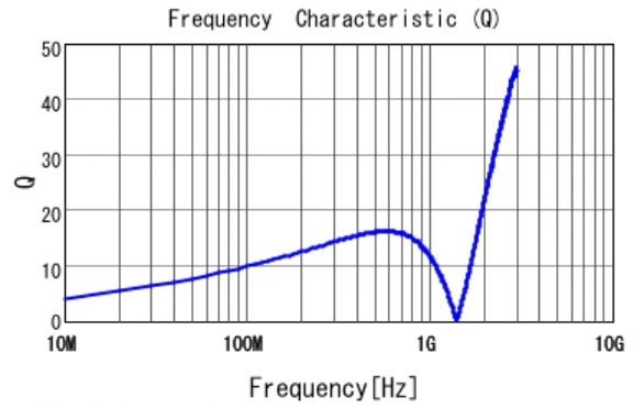
■ LQG15HN56NG02 Q
