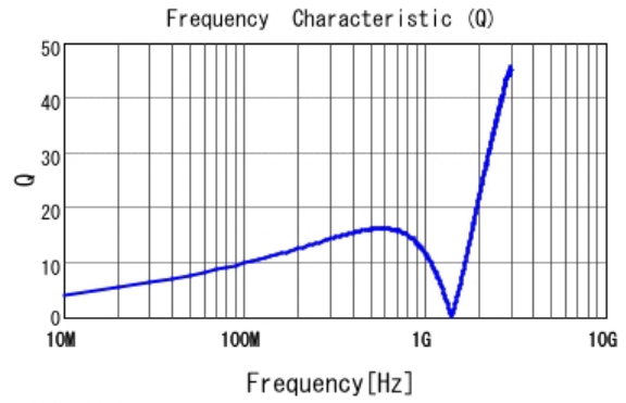
■ LQG15HN56NJ02 Q
