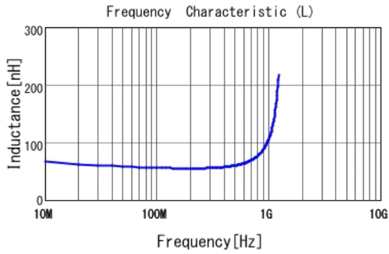
■ LQG15HN56NJ02 L
