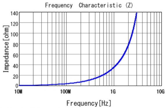
■ LQG15HN5N6S02 |Z|
