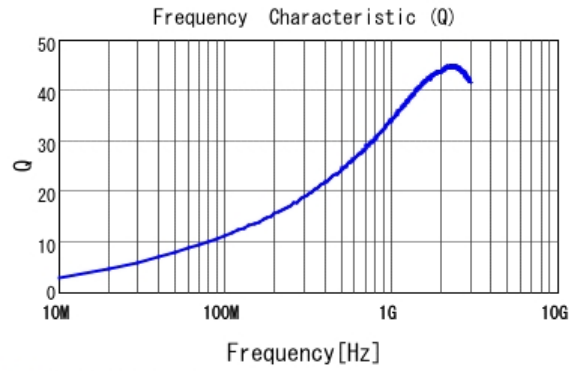
■ LQG15HN5N6S02 Q
