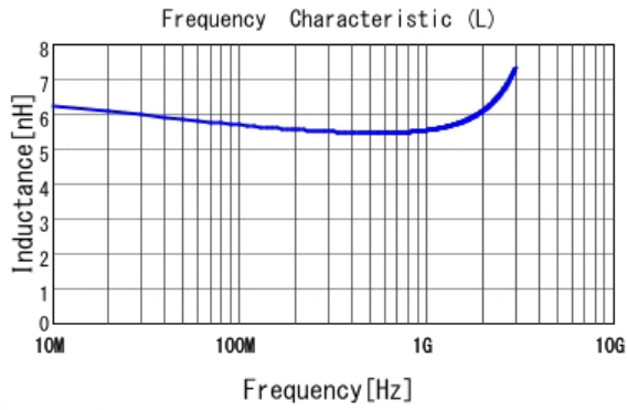
■ LQG15HN5N6S02 L
