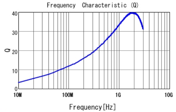
■ LQG15HN6N2S02 Q
