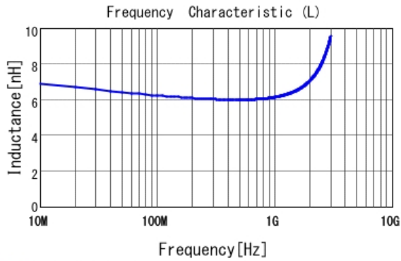
■ LQG15HN6N2S02 L
