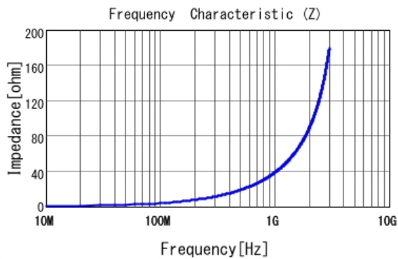
■ LQG15HN6N2S02 |Z|
