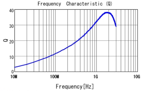
■ LQG15HN6N8J02 Q
