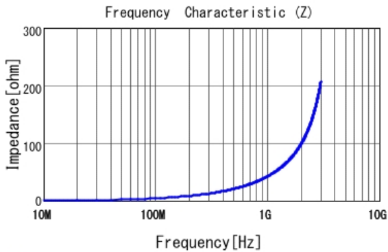
■ LQG15HN6N8J02 |Z|
