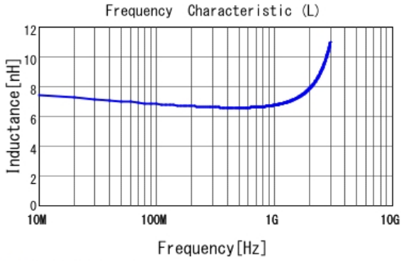
■ LQG15HN6N8J02 L
