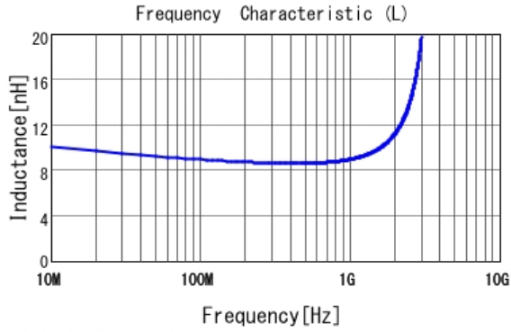
■ LQG15HN9N1J02 L
