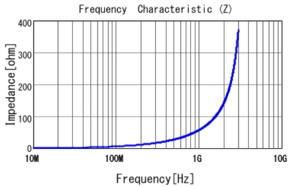
■ LQG15HN9N1J02 |Z|
