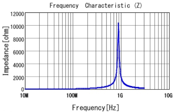
■ LQG15HNR10J02 |Z|
