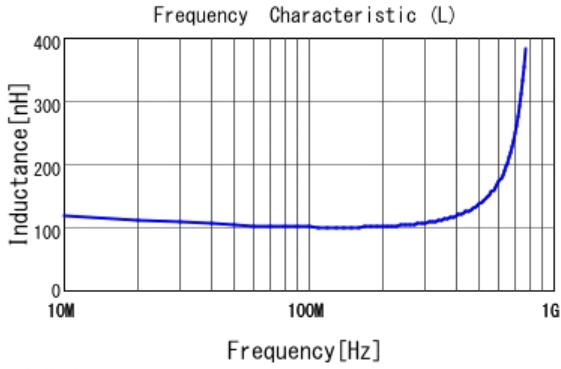
■ LQG15HNR10J02 L
