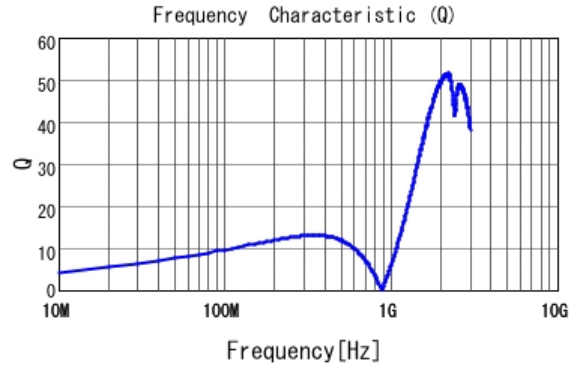
■ LQG15HNR10J02 Q
