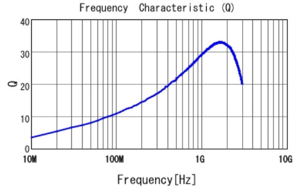
■ LQG15HS10NJ02 Q
