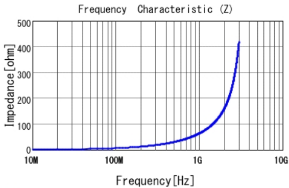
■ LQG15HS10NJ02 |Z|
