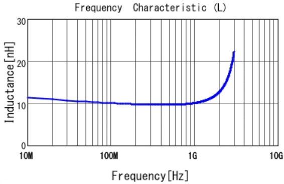
■ LQG15HS10NJ02 L
