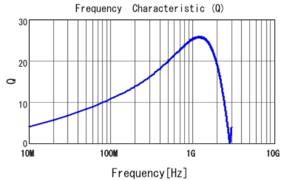
■ LQG15HS15NH02 Q
