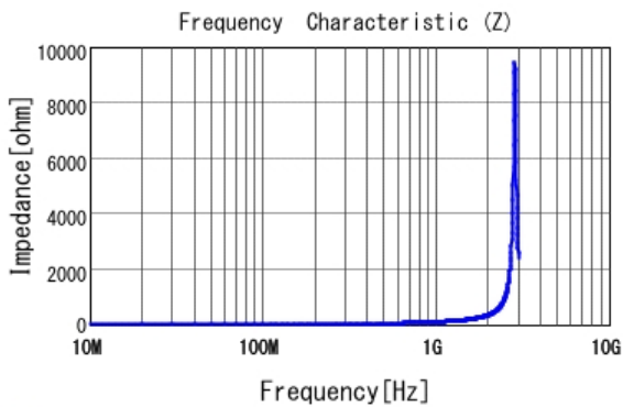
■ LQG15HS15NH02 |Z|
