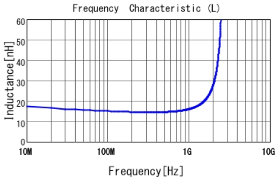
■ LQG15HS15NH02 L
