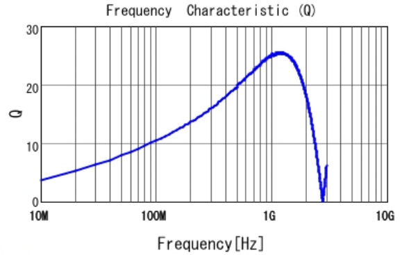
■ LQG15HS18NJ02 Q
