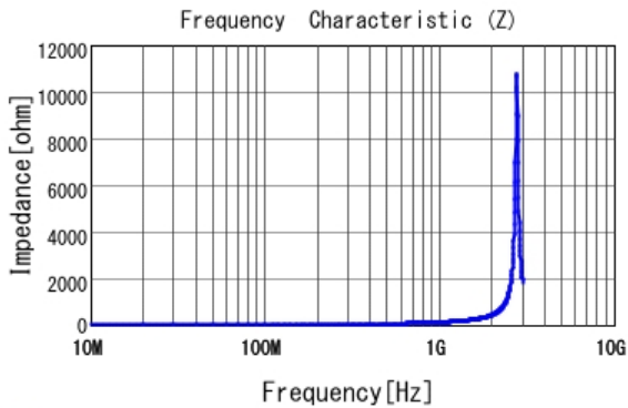
■ LQG15HS18NJ02 |Z|
