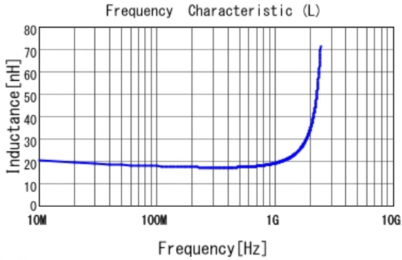
■ LQG15HS18NJ02 L
