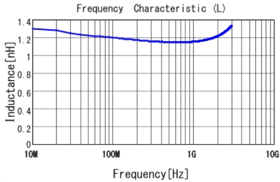
■ LQG15HS1N2B02 L
