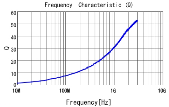
■ LQG15HS1N2B02 Q
