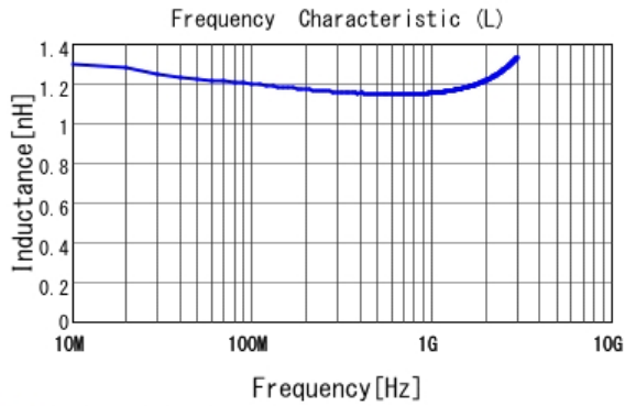
■ LQG15HS1N2S02 L
