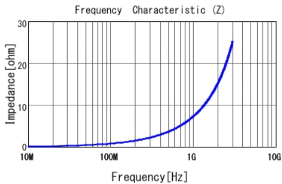
■ LQG15HS1N2S02 |Z|
