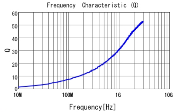
■ LQG15HS1N2S02 Q
