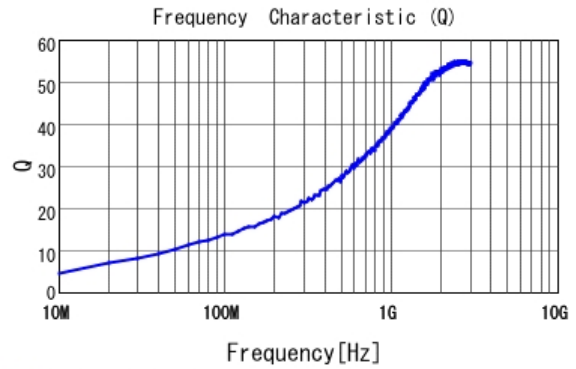
■ LQG15HS1N3S02 Q
