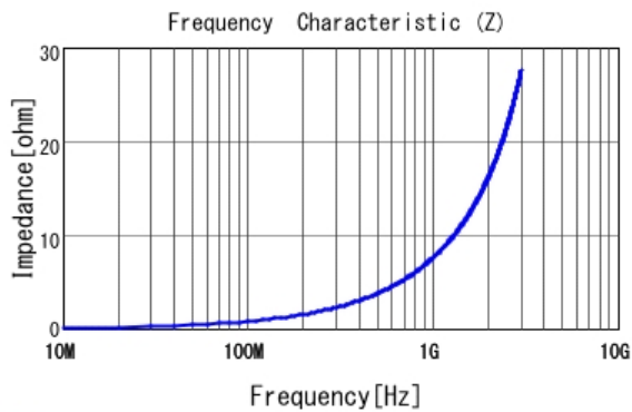
■ LQG15HS1N3S02 |Z|
