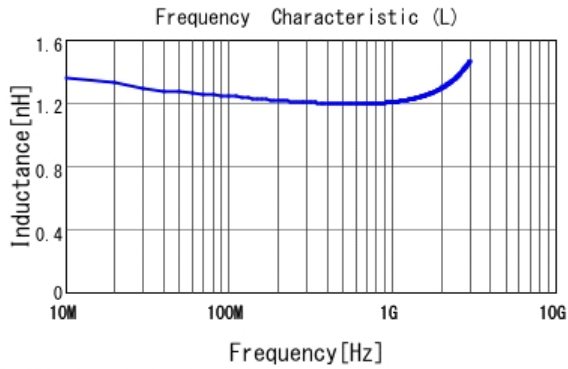
■ LQG15HS1N3S02 L
