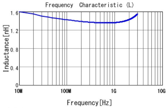
■ LQG15HS1N5S02 L
