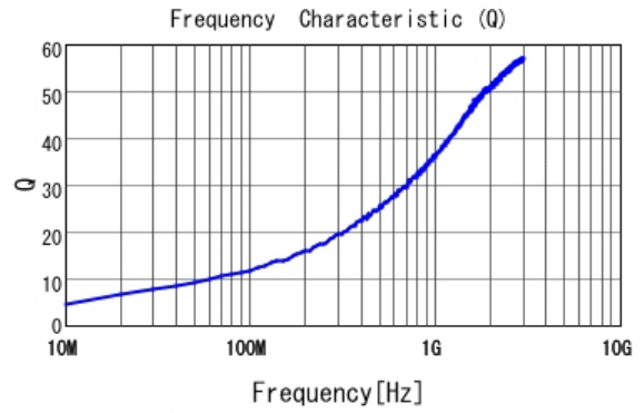
■ LQG15HS1N5S02 Q
