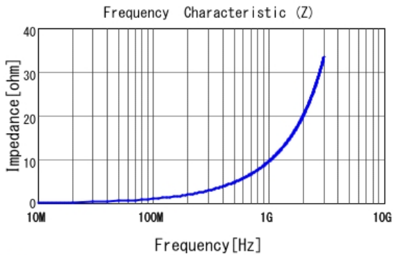
■ LQG15HS1N6S02 |Z|
