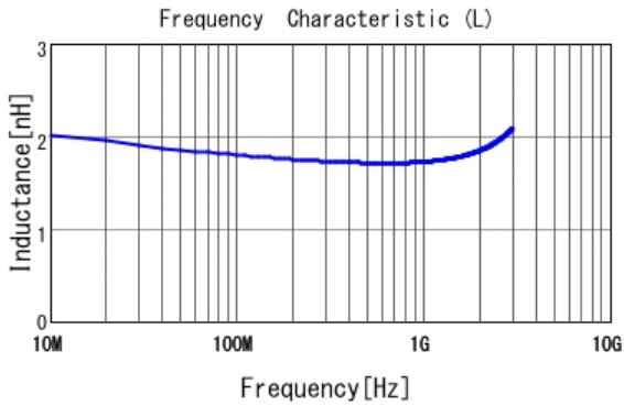
■ LQG15HS1N8S02 L
