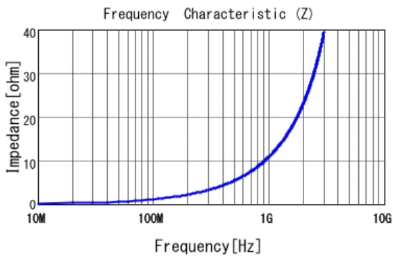
■ LQG15HS1N8S02 |Z|
