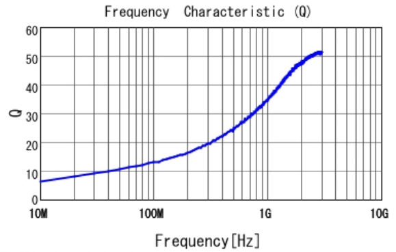
■ LQG15HS1N8S02 Q
