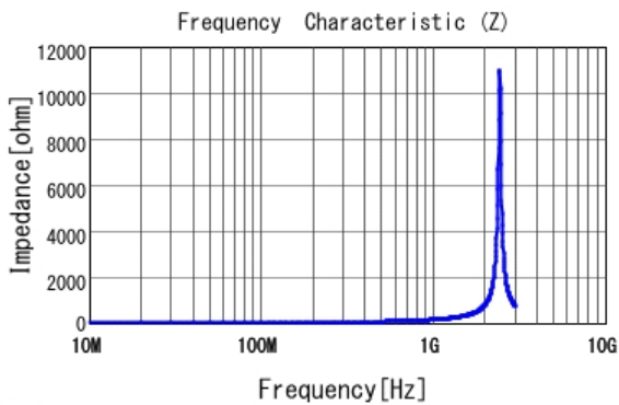
■ LQG15HS22NJ02 |Z|
