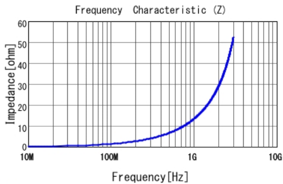
■ LQG15HS2N2B02 |Z|
