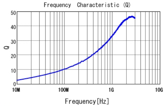
■ LQG15HS2N2B02 Q
