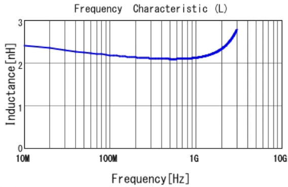
■ LQG15HS2N2B02 L
