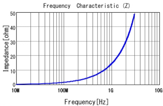
■ LQG15HS2N4S02 |Z|
