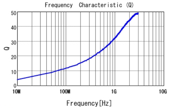
■ LQG15HS2N7B02 Q
