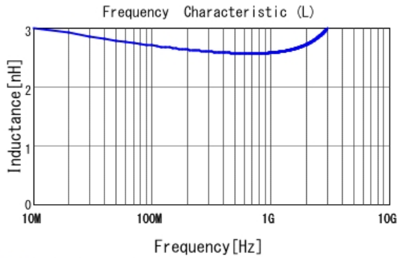
■ LQG15HS2N7B02 L
