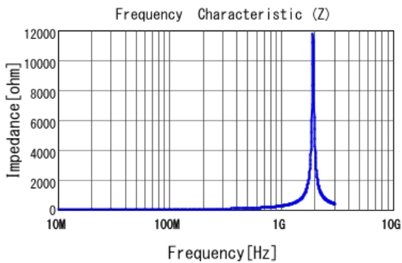
■ LQG15HS33NJ02 |Z|
