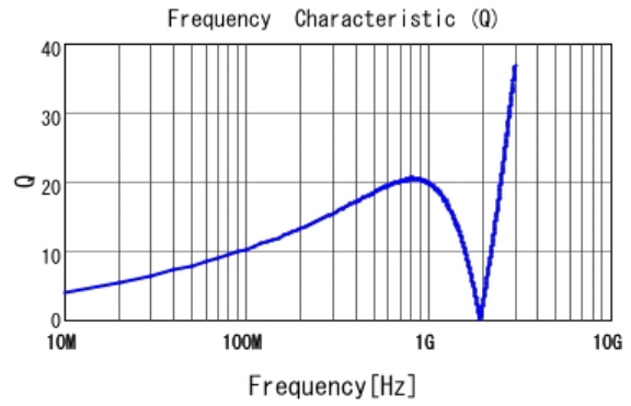
■ LQG15HS33NJ02 Q
