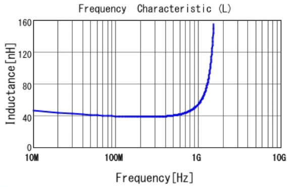
■ LQG15HS39NJ02 L
