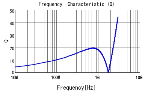
■ LQG15HS39NJ02 Q
