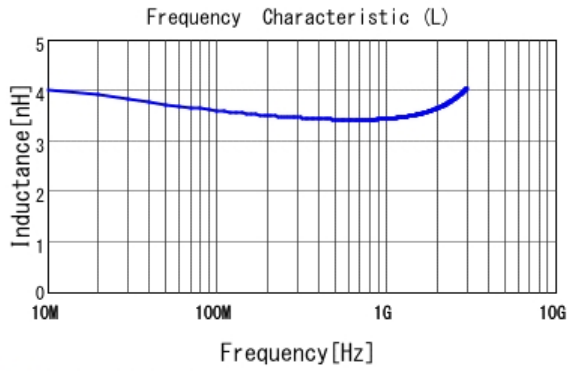
■ LQG15HS3N6S02 L
