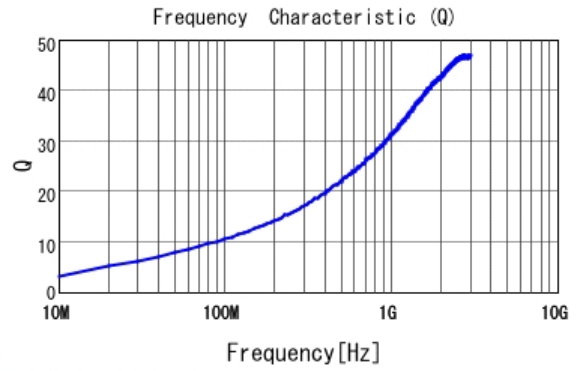
■ LQG15HS3N6S02 Q
