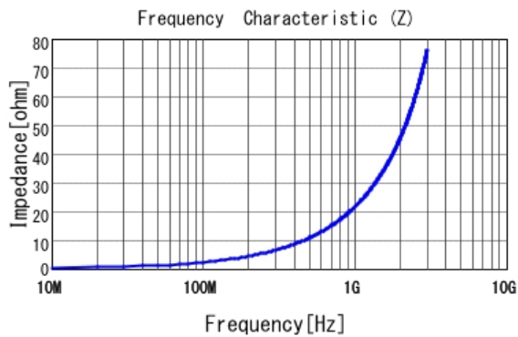
■ LQG15HS3N6S02 |Z|
