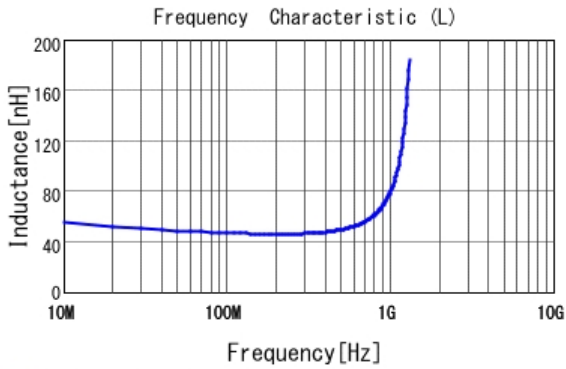
■ LQG15HS47NJ02 L
