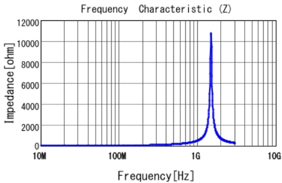
■ LQG15HS47NJ02 |Z|
