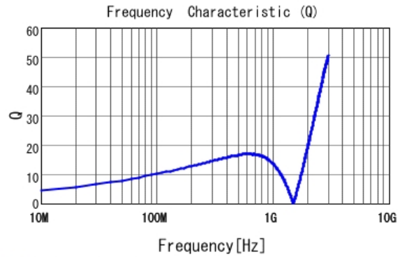
■ LQG15HS47NJ02 Q
