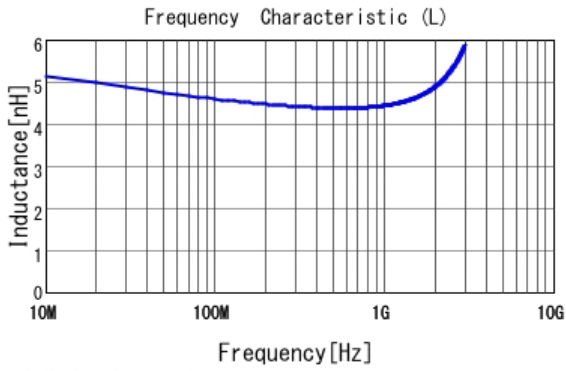
■ LQG15HS4N7B02 L
