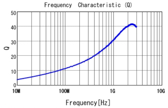
■ LQG15HS4N7B02 Q
