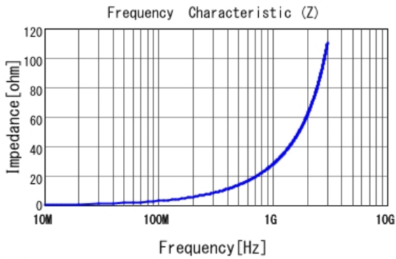
■ LQG15HS4N7B02 |Z|
