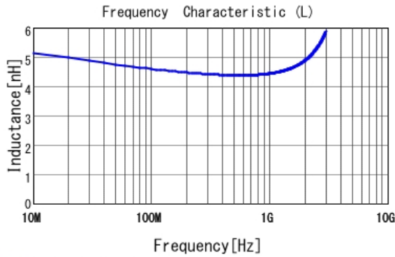
■ LQG15HS4N7S02 L
