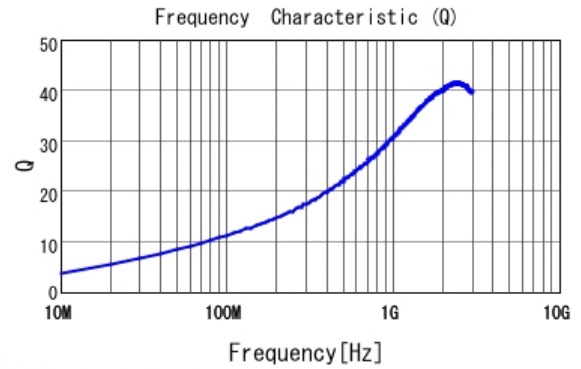
■ LQG15HS4N7S02 Q
