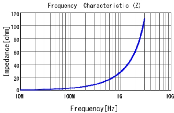
■ LQG15HS4N7S02 |Z|
