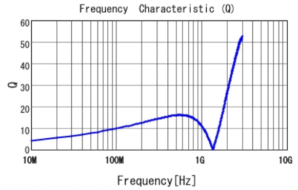
■ LQG15HS56NJ02 Q
