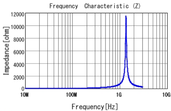
■ LQG15HS56NJ02 |Z|
