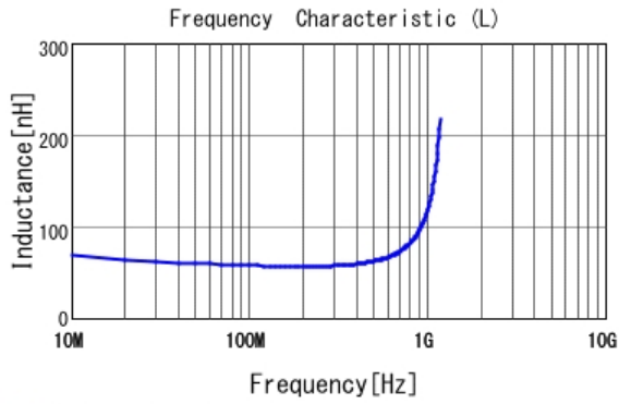
■ LQG15HS56NJ02 L
