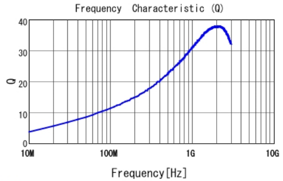
■ LQG15HS5N6B02 Q
