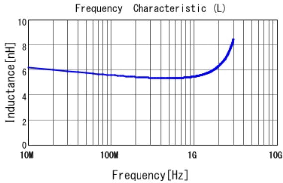
■ LQG15HS5N6B02 L
