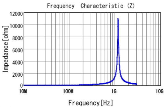
■ LQG15HS68NJ02 |Z|
