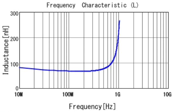
■ LQG15HS68NJ02 L
