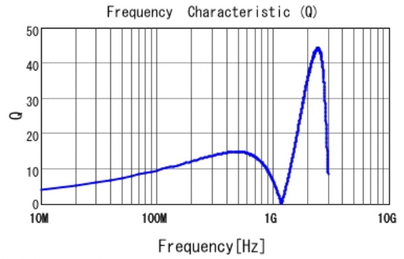
■ LQG15HS68NJ02 Q
