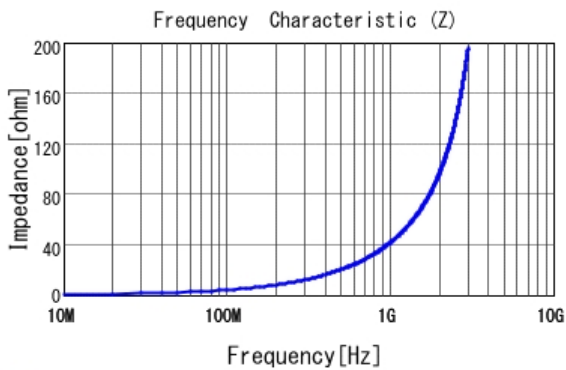
■ LQG15HS6N8G02 |Z|
