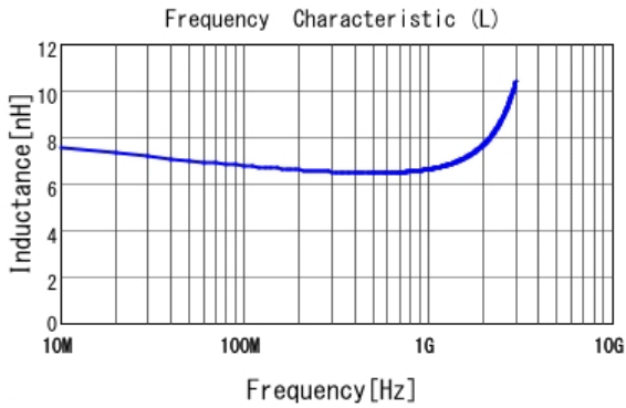
■ LQG15HS6N8G02 L
