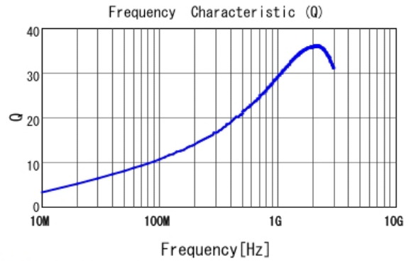
■ LQG15HS6N8G02 Q
