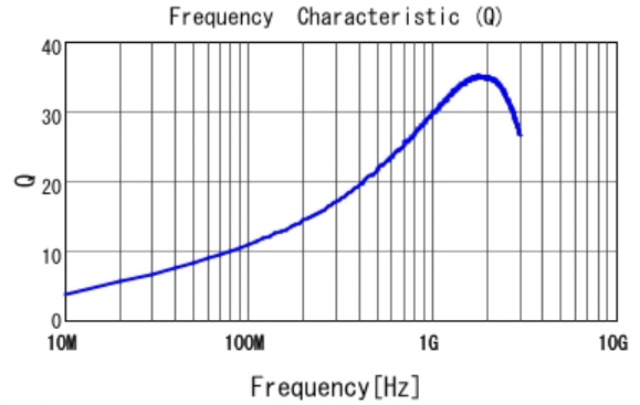
■ LQG15HS7N5J02 Q
