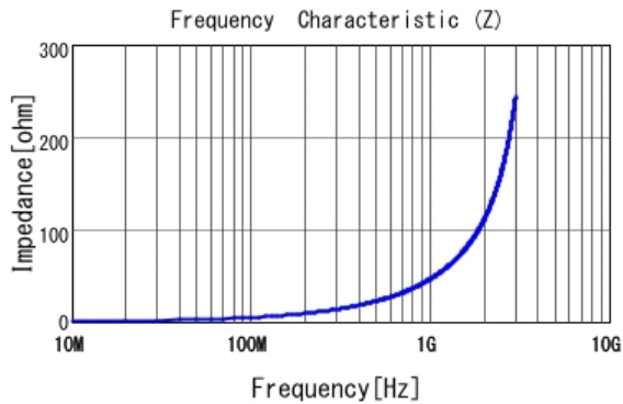
■ LQG15HS7N5J02 |Z|
