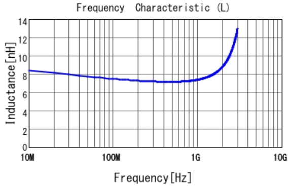
■ LQG15HS7N5J02 L
