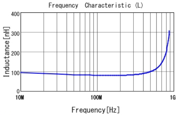
■ LQG15HS82NJ02 L
