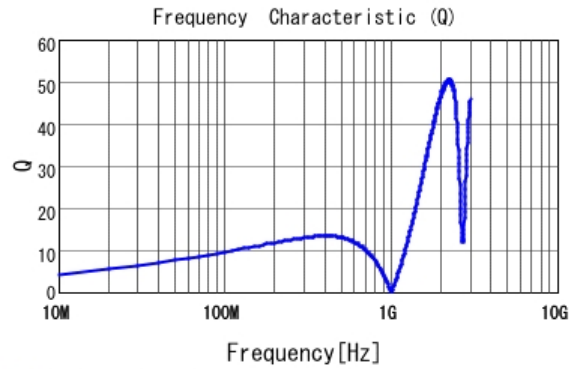
■ LQG15HS82NJ02 Q
