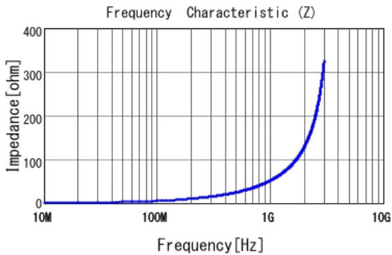
■ LQG15HS8N2J02 |Z|
