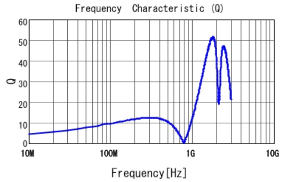
■ LQG15HSR12J02 Q
