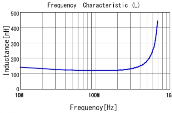
■ LQG15HSR12J02 L
