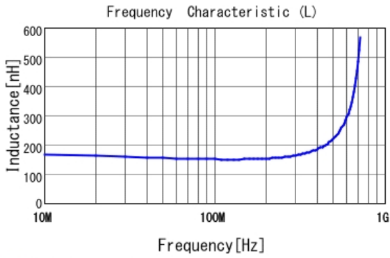
■ LQG15HSR15J02 L
