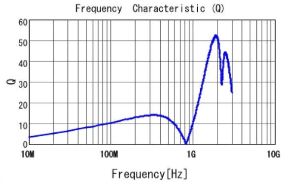
■ LQG15HSR15J02 Q
