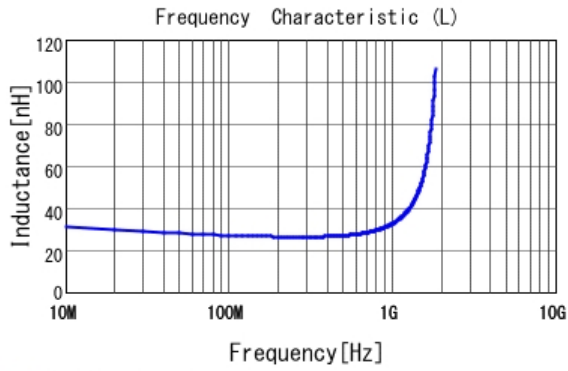
■ LQG15HZ27NJ02 L
