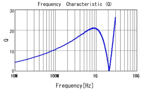
■ LQG15HZ27NJ02 Q
