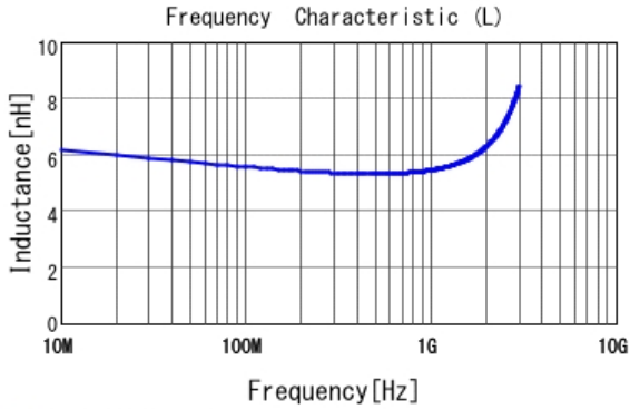
■ LQG15HZ5N6B02 L
