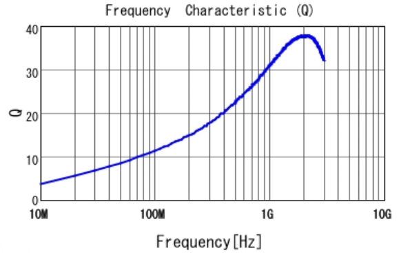
■ LQG15HZ5N6B02 Q
