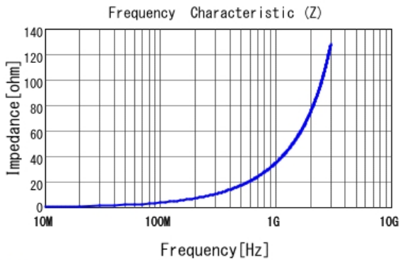
■ LQG15WH5N6S02 |Z|
