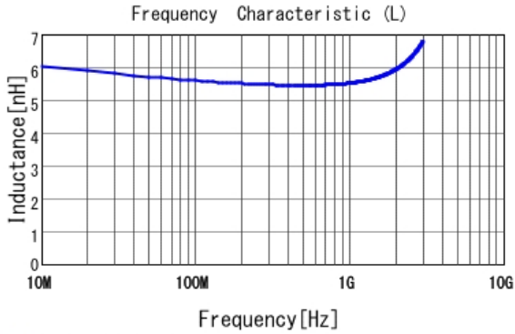
■ LQG15WH5N6S02 L
