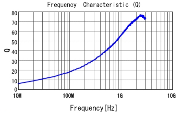
■ LQG15WH5N6S02 Q
