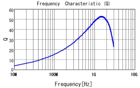
■ LQG18HN10NJ00 Q
