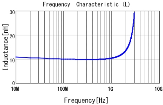
■ LQG18HN10NJ00 L
