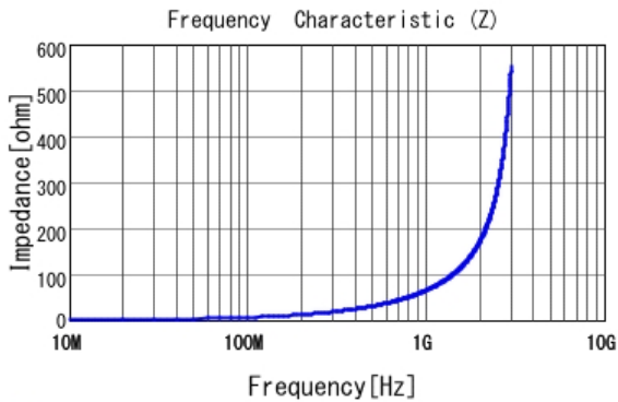
■ LQG18HN10NJ00 |Z|
