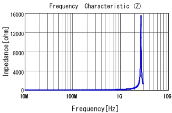
■ LQG18HN18NJ00 |Z|
