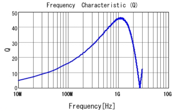
■ LQG18HN18NJ00 Q
