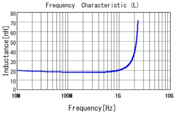
■ LQG18HN18NJ00 L
