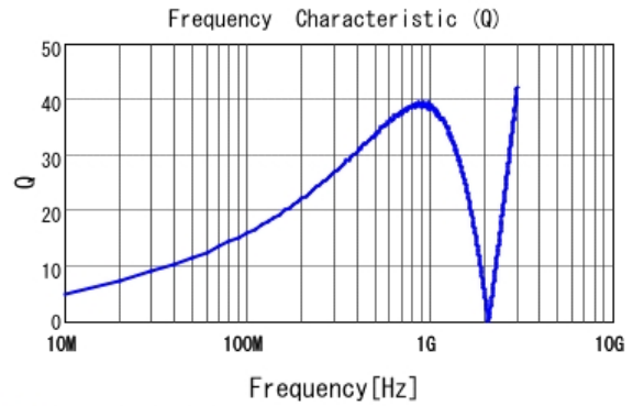
■ LQG18HN27NJ00 Q
