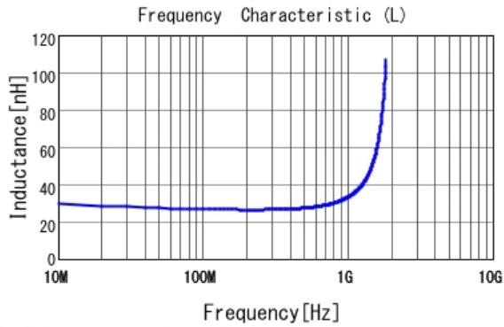
■ LQG18HN27NJ00 L
