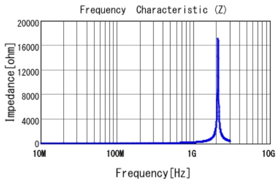
■ LQG18HN27NJ00 |Z|
