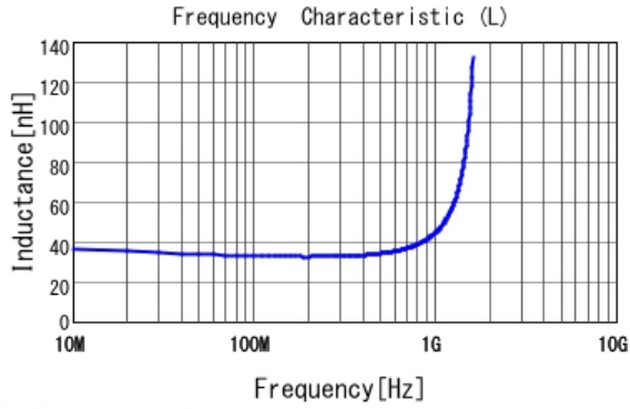
■ LQG18HN33NJ00 L
