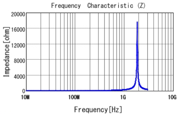
■ LQG18HN33NJ00 |Z|
