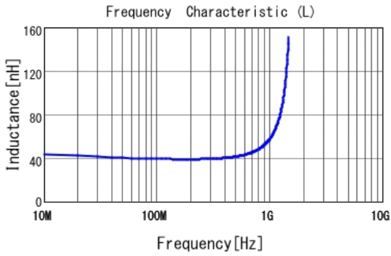
■ LQG18HN39NJ00 L
