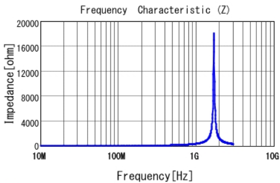
■ LQG18HN39NJ00 |Z|
