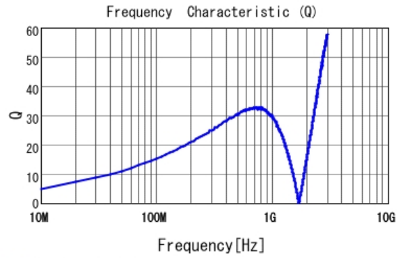
■ LQG18HN39NJ00 Q
