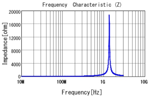
■ LQG18HN56NJ00 |Z|
