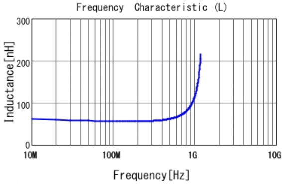
■ LQG18HN56NJ00 L
