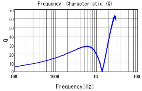
■ LQG18HN56NJ00 Q
