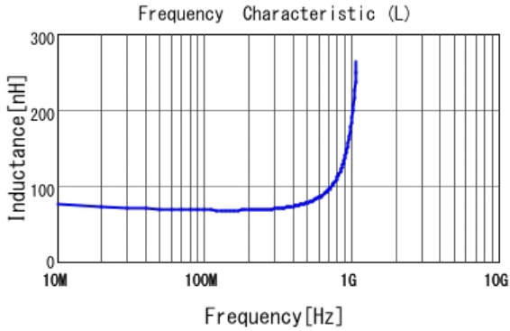
■ LQG18HN68NJ00 L
