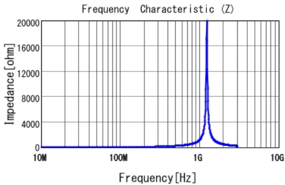
■ LQG18HN68NJ00 |Z|
