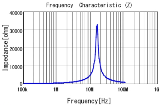
■ LQH3NPN470MME |Z|
