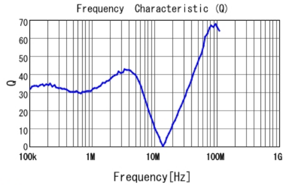
■ LQH5BPN220M38 Q
