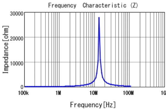
■ LQH5BPN220M38 |Z|
