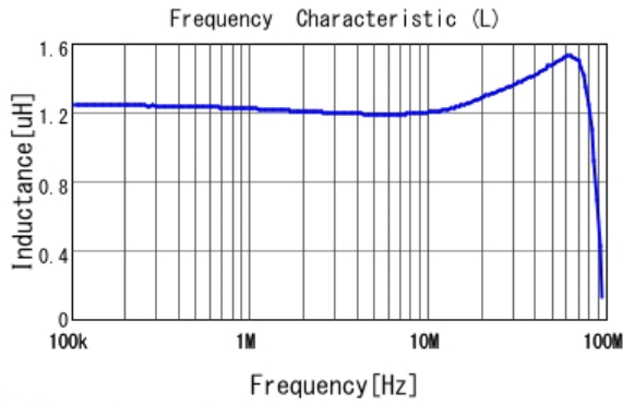
■ LQM21PN1R0NGC L
